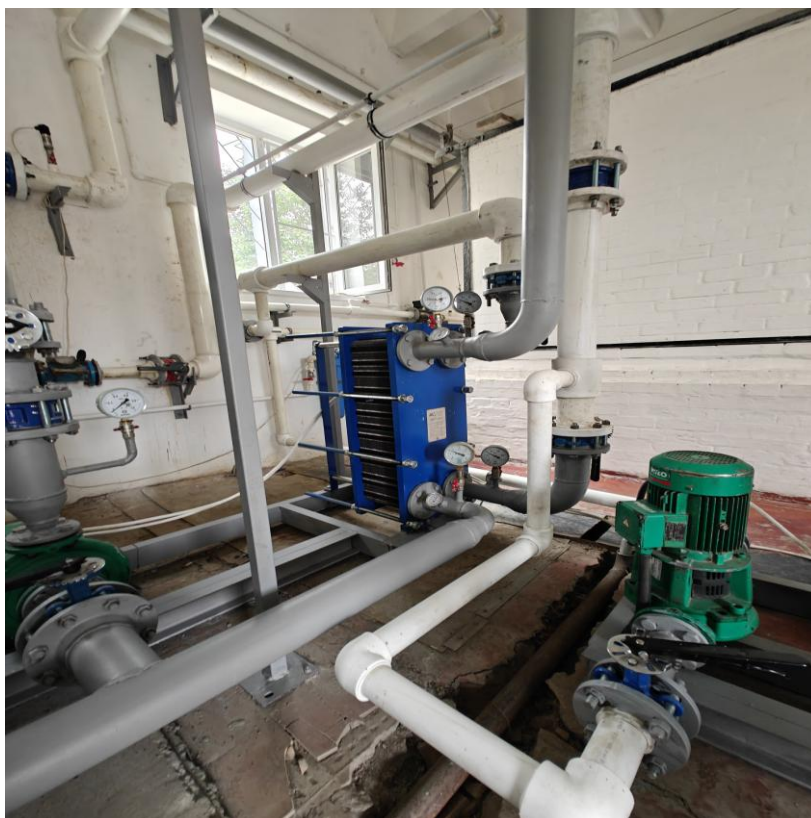
Реконструкция системы горячего водоснабжения на котельной пер.17 Новый,5-1
